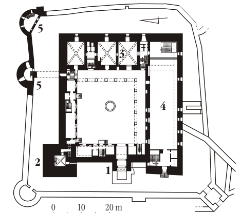
Plan przyziemia zamku – stan obecny rys. wg M. Ciborowskiego
